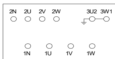
Slika 0-1: razporeditev priključkov na pokrovu transformatorja
