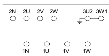
Slika 4-1: razporeditev priključkov na pokrovu transformatorja
